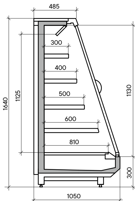
CRETE H-1600 DG
